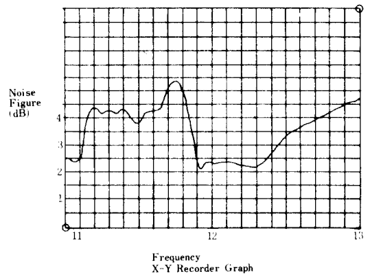
(c) 증폭기의 잡음지수 Amplifier noise figure.
