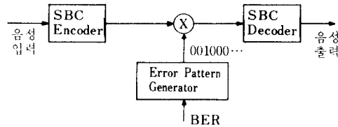
그림 8 비트에러 시뮬레이션블록선도 Block diagram for the bit error simulation.
