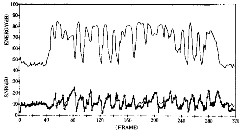
그림 9 단시간 에너지대 SNR (전송율 : 16Kbps) — : no error -▲- : BER = 10 -3 (a) 음성 1 (남성) (b) 음성 2 (여성) Short-time energy vs SNR (bit rate: 16 Kbps) — : no error -▲- : BER = 10 -3 (a) Speech 1 (male) (b) Speech 2 (female).
