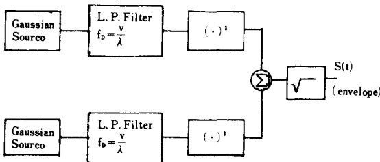
그림 3 레일리 페이딩 채널 시뮬레이터블록선도 Block diagram of the Rayleigh fading channel simulator.
