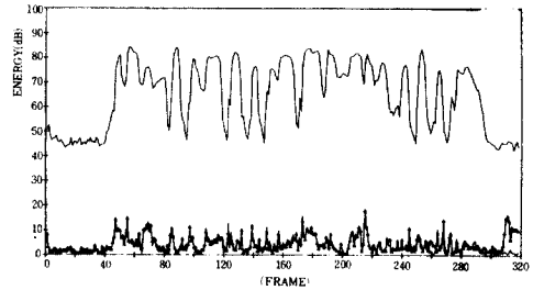
그림 10 단시간 에너지 대 LPC 거리 척도 (전송율 : 16 Kbps) — : no error -▲- : BER = 10 -3 (a) 음성 1 (남성) (b) 음성 2 (여성) Short-time energy vs LPC distance measurement (bit rate: 16 Kbps) (a) Speech 1 (male) (b) Speech 2 (female).
