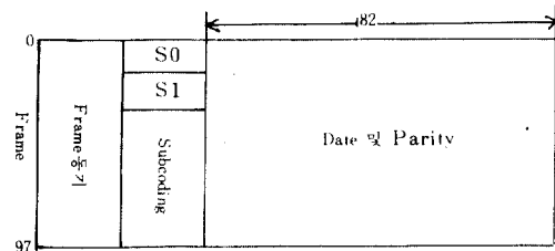
그림 3 서브코드 프레임형식 Subcode frameformat.
