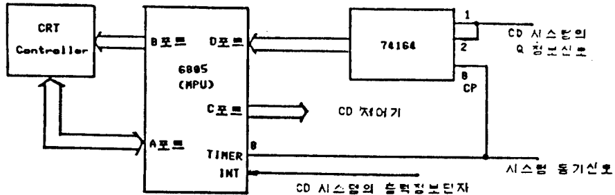
그림16 DAS 제어기 블록회로도 DAS controller block diagram.
