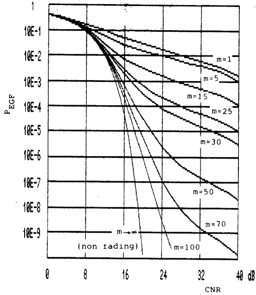
그림 5. 페이딩 채널상에서 가우스성 잡음의 영향을 받는 4-레벨 ASK 신호의 오류특성 Error rate characteristic of 4-level ASK signal influenced by Gaussian noise in fading channel.
