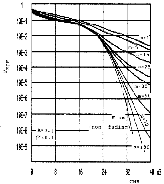
그림 8. 페이딩 채널상에서 임펄스성 잡음의 영향을 받는 16 QAM 신호의 오류특성 Error rate characteristic of 16 QAM signal influenced by Impulsive noise in fading channel.
