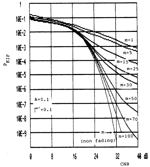
그림 6. 페이딩 채널상에서 임펄스성 잡음의 영향을 받는 4-레벨 ASK 신호의 오류특성 Error rate characteristic of 4-level ASK signal influenced by Impulsive noise in fading channel.
