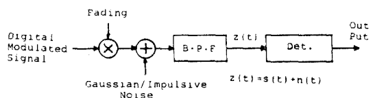
그림 1. 일반적인 해석모델 Generalized analysis model.
