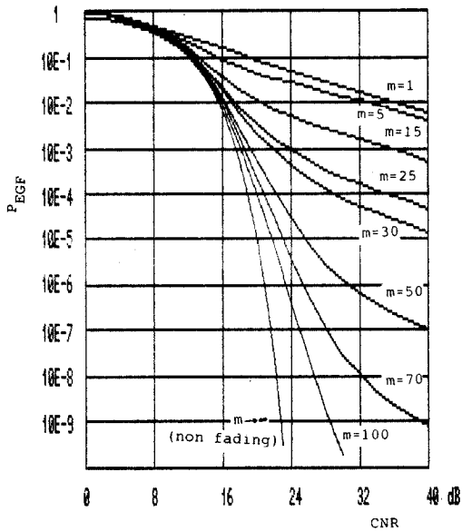
그림 7. 페이딩 채널상에서 가우스성 잡음의 영향을 받는 16 QAM 신호의 오류특성 Error rate characteristic of 16 QAM signal influenced by Gaussian noise in fading channel.
