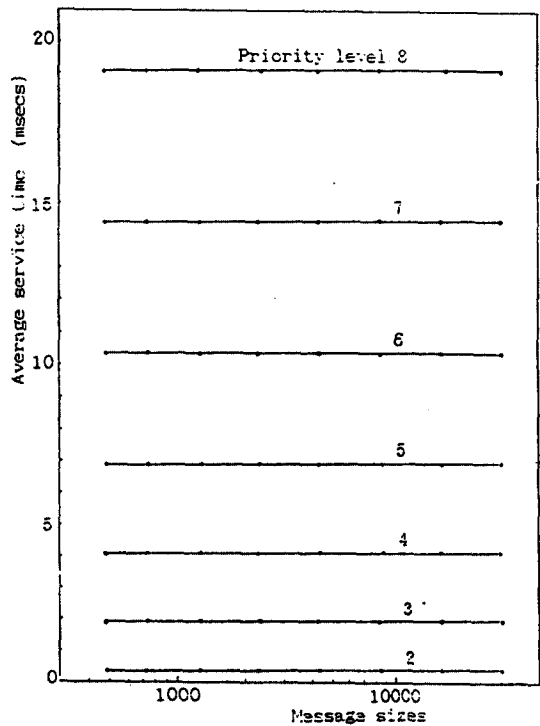
그림 2. 메시지 크기에 따른 평균에 매체 이용시간 Average service times on message sizes.
