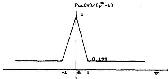
그림 5b. GF(5)에서 非二元 GMW 부호계열의 해밍자기상관 함수 특성 Hamming autocorrelation function characteristics of non-binary GMW code sequence over GF(5).
