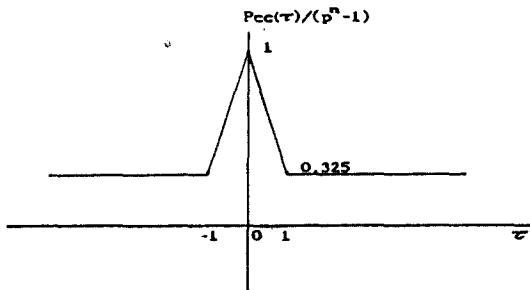
그림 5a. GF(3)에서 非二元 GMW 부호계열의 해밍자기상관 함수 특성 Hamming autocorrelation function characteristics of non-binary GMW code sequence over GF(3).
