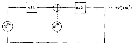
그림 3. GF(3)에서 GF(3 4 )의 m-계열발생기 M sequence generator of GF(3 4 ) over GF(3 2 )
