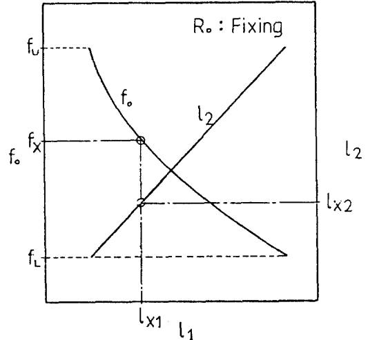
그림 3. 공진주파수와 장하 리액턴스와의 관계 ( X_i = Z_0 \tan(kl_i) , i=1,2 ).
