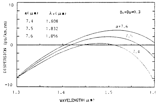
그림 2. a의 변화에 대한 이중형 코어(DSC) W형 광섬유의 총분산 변화 Fig.2. Relationship between wavelength and total dispersion for different values of core radius a ( \Delta_1=0.35\% , \rho=1.6 , C=1.2 , \alpha=2 )
