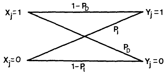
그림 11. 결정 전이 확률 Fig. 11. Transition Probability for the Hard Decision Channel
