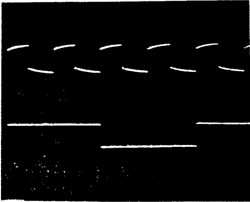
(a) 표분클럭 합성부에 가해진 시스템클럭( f_c : 상)과 최대 합성초기치(3FFFFFF hex )에의 합성된 표분클럭( f_m : 하) Synthesized sampling clock(up) by the system clock (down) in clock synthesizing part
