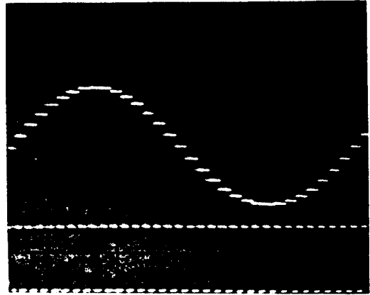
(b) 표분클럭( f_m : 하)으로 만들어진 정현출력파형( f_o : 상) Sinusoidal output waveform(up) by the synthesized sampling clock(down)
