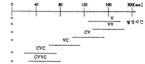
그림 6. 유성선호의 발생시간
