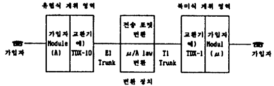
그림 1. 북미 / 유럽 전송방식간 연동계획
