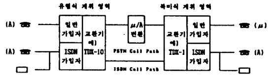
그림 3. 트렁크의 분리
