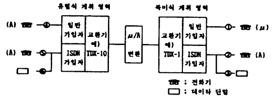
그림 2. ISDN 망구조
