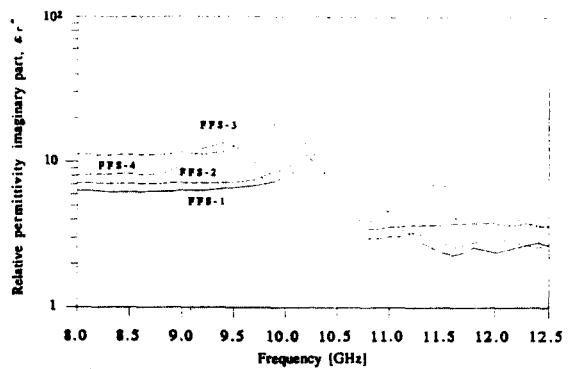
그림 7. 페라이트-탄화규소 복합물의 비유전율 허수성분( \epsilon_r'' ) 스펙트럼
