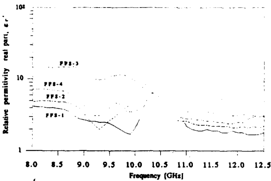
그림 6. 페라이트-탄화규소 복합물의 비유전율 실수성분( \epsilon_r' ) 스펙트럼
