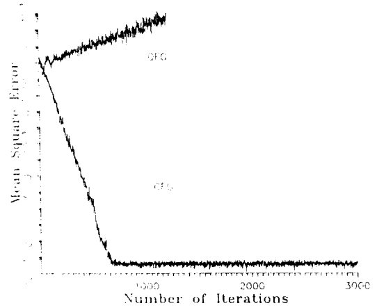
그림 8. \alpha_1=0.5, \alpha_2=0.5 를 가진 QFG 및 \alpha_1=0.5, \alpha_2=0.5, \alpha_3=-0.1 를 가진 CFG에 대한 MSE 학습 곡선 (VI) Fig 8. MSE learning curves for the QFG with \alpha_1=0.5 and \alpha_2=0.5 , and CFG with \alpha_1=0.5, \alpha_2=0.5, \alpha_3=-0.1 (VI)
