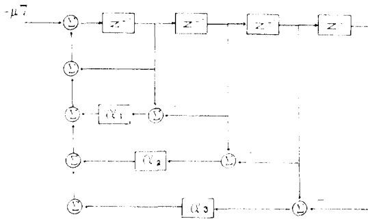
그림 1. CFG 알고리즘의 구조 Fig 1. The structure of the CFG algorithm
