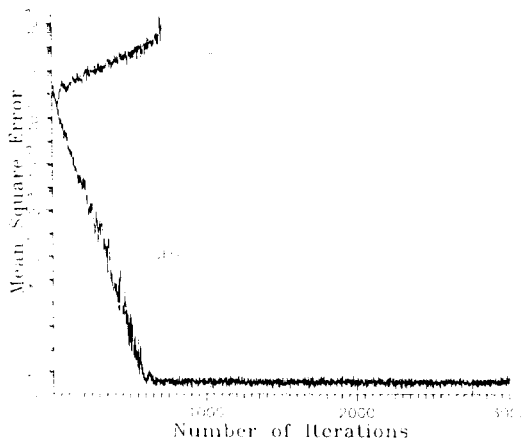
그림 6. \alpha_1=1 를 가진 LFG 및 \alpha_1=1, \alpha_3=-0.06 를 가진 CFG에 대한 MSE 학습 곡선 (IV) Fig 6. MSE learning curves for the LFG with \alpha_1=1 and CFG with \alpha_1=1 and \alpha_3=-0.06 (IV)
