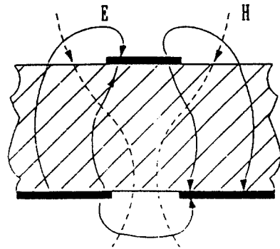
(b) 기모드인 경우의 전계 및 자계 분포
