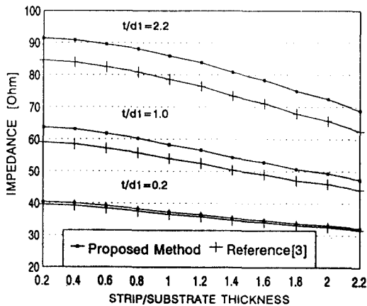
그림 3-4. 마이크로스트립-슬롯 결합선로의 기모드에 대한 특성임피던스
