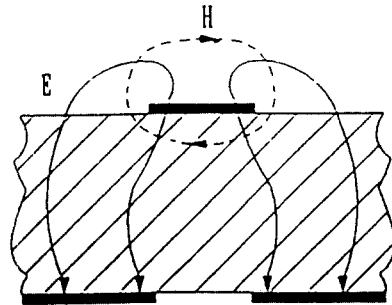
(a) 우모드인 경우의 전계 및 자계 분포
