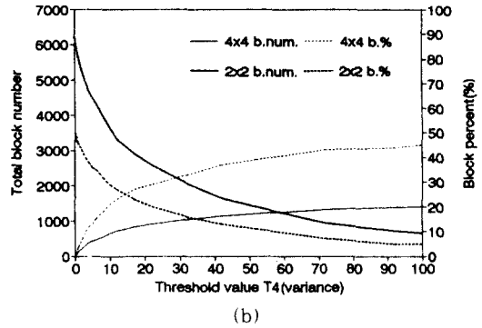
그림 8. 임계치 T_4 의 증가에 따른 방법 2의 성능 (a) 평균 전송율과 PSNR (b) 전송되는 블록 수와 백분율
