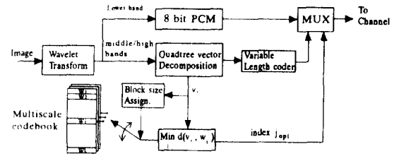
그림 3. BWT 영상의 부호화 시스템 Fig 3. Full encoding system of the BWT image
