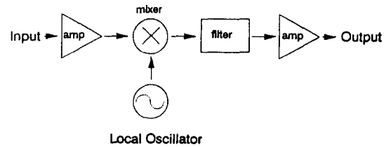
그림 8. 주파수 변환기 블록도 Fig. 8. Block diagram of frequency converter
