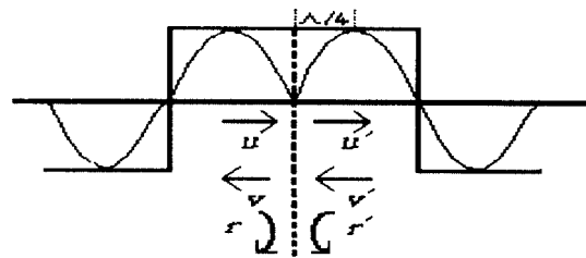
그림 6. \lambda/4 phase shifted DFB-LD의 중심에서의 회절격자의 구조 및 위상 Fig. 6. The schematic diagram and the phase of the grating to \lambda/4 phase shifted DFB-LD center
