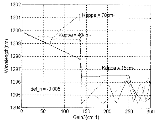
그림 8. Coupling 상수에 따른 tuning trend(연속적인 위상을 가지는 3전극 DFB-LD) Fig. 8. The tuning trend about a coupling coefficient(The three section DFB-LD with a continuous phase)
