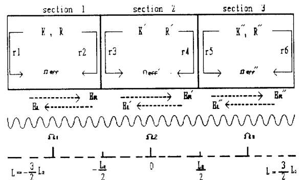
그림 2. 연속적인 위상을 갖는 3전극 DFB 구조 Fig. 2. The three section DFB-LD schematic diagram with a continuous phase
