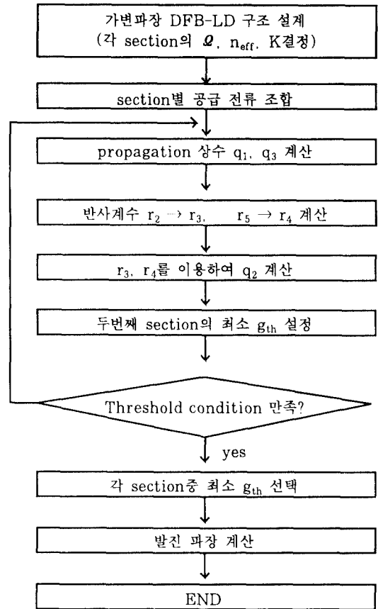
그림 4. 3전극 가변파장 DFB-LD의 발광파장을 구하기 위한 flow chart
