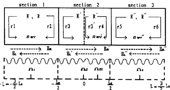
그림 5. \lambda/4 phase-shifted 3전극 DFB-LD 구조 Fig. 5. The \lambda/4 phase-shifted three section DFB-LD schematic diagram
