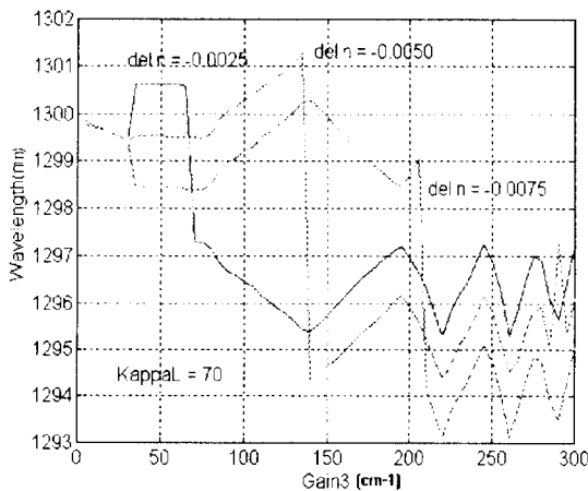
그림 7. \Delta n_2 의 변화에 따른 tuning trend(연속적인 위상을 가지는 3전극 DFB-LD) Fig. 7. The tuning trend about a change of \Delta n_2 (The three section DFB-LD with a continuous phase)
