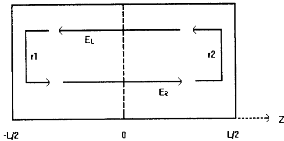
그림 1. 단면 반사계수 r_1 과 r_2 를 가지는 길이 L 인 one section DFB레이저의 schematic diagram Fig. 1. The schematic diagram of one section DFB-LD with facet reflection coefficient r_1, r_2 .
