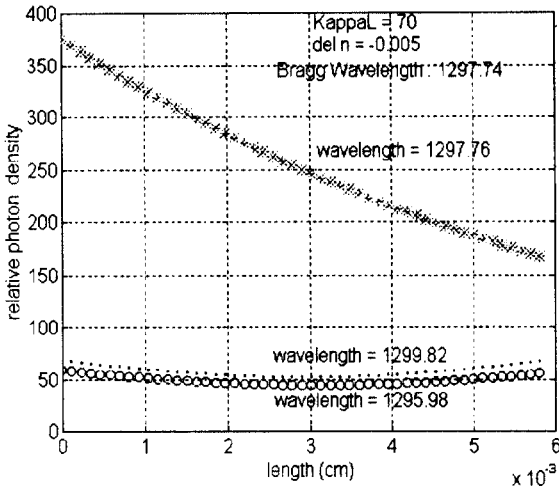
그림 11. 길이에 따른 photon density의 변화 Fig. 11. The change of photon density to length
