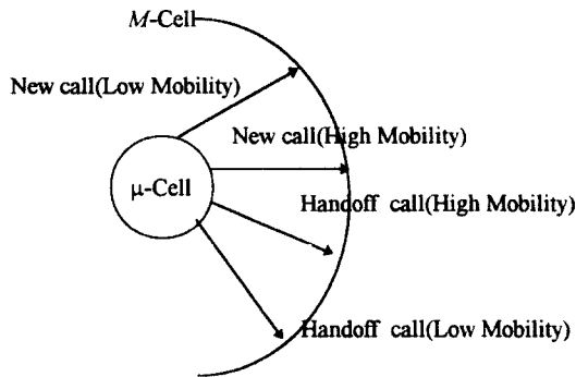
그림 2 중첩셀 구조에서 계층간 트래픽 흐름도 Fig. 2 Overflowed Traffic transfer between Micro/Macro cell
