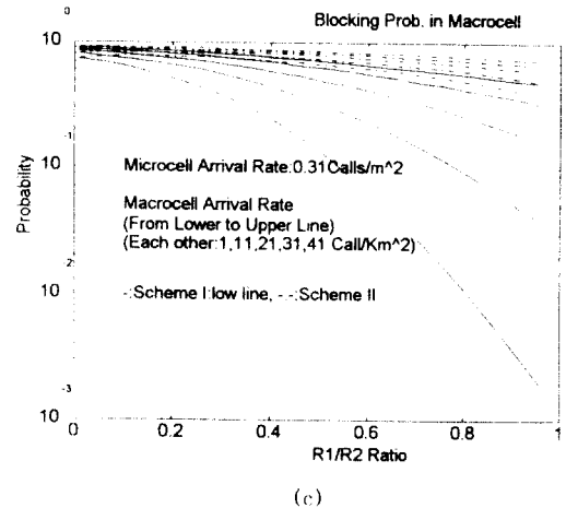
그림 8. 소프트 핸드오프 영역에 따른 매크로셀의 블러킹 확률 분포(방식 I, II)
