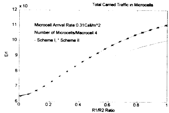
그림 12. 마이크로 셀에서 처리하는 트래픽량 Fig. 12 Carried Traffic of microcell
