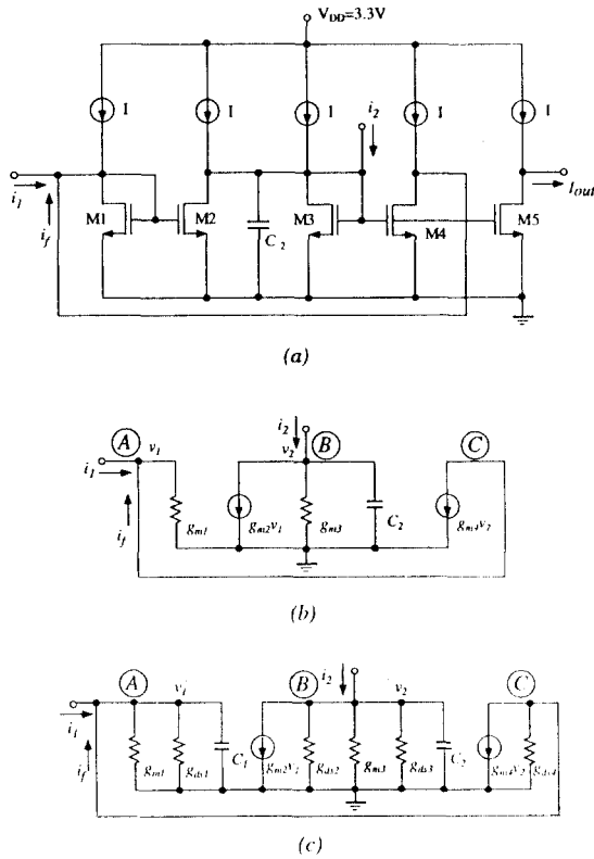
그림 1. 연속시간 전류모드 CMOS 적분기. (a) 회로 구조 (b) 1차 소신호 등가회로 (c) 2차 소신호 등가회로 Fig. 1. Continuous-time current-mode CMOS integrator (a) Architecture (b) First-order small signal equivalent circuit (c) Second-order small signal equivalent circuit
