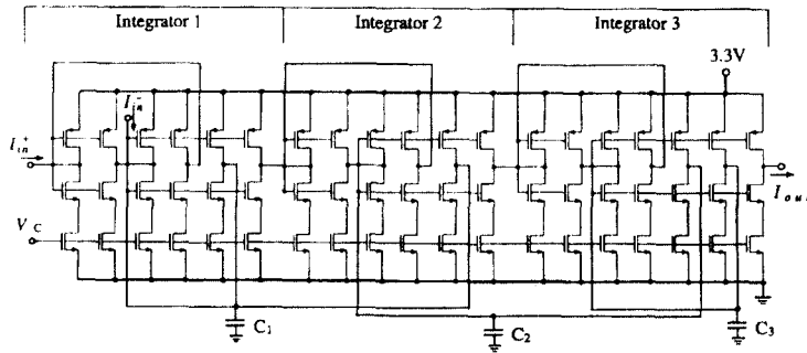
그림 4. 설계된 전류모드 3차 능동 저역통과 필터 Fig. 4. Designed current-mode 3rd-order active lowpass filter
