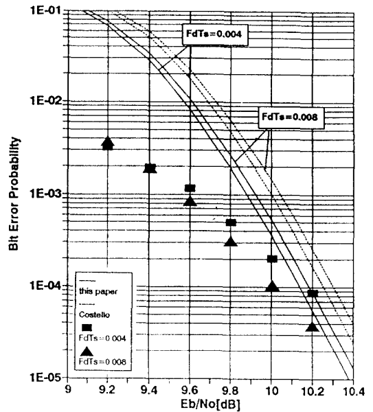
그림 6. 레일리 페이딩 채널에서 RS/Trellis 연결 부호변조 시스템의 비트오율 (63, 47)RS + TCM( r = 2/3, \mu = 6 ). Fig. 6 The bit error probability of RS/Trellis concatenated code-modulation system in the Rayleigh fading channel, (63, 47)RS + TCM( r = 2/3, \mu = 6 ).
