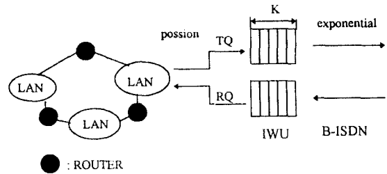
그림 8. IWU의 모델링
