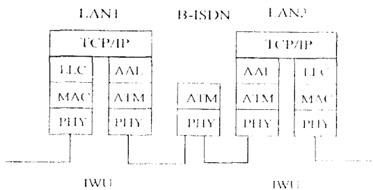
그림 1. 망의 상호 연결을 위한 프로토콜 구조
