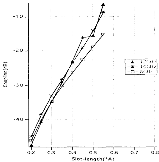
그림 8. 슬롯 길이에 따른 결합특성 변화 Fig. 8 Coupling versus slot length ( X_{p1} = X_{p2} = X_{s1} = X_{s2} = A/4 , W = 0.072\lambda , t = 0.05\text{ in.} )
