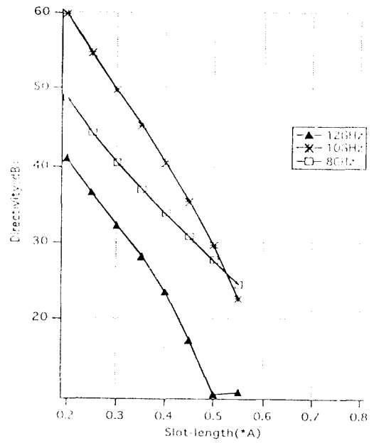
그림 9. 슬롯 길이에 따른 방향성 변화 Fig. 9 Directivity versus slot length ( X_{p1} = X_{p2} = X_{s1} = X_{s2} = A/4 , W = 0.072\lambda , t = 0.05\text{ in.} )
