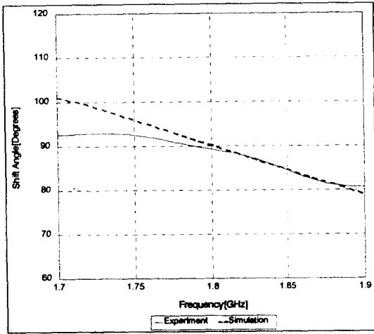
(c) 90° 위상천이기
