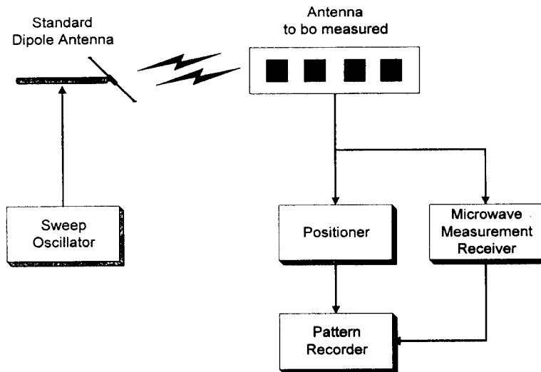
그림 5. 안테나의 방사패턴 측정 시스템의 구성도
