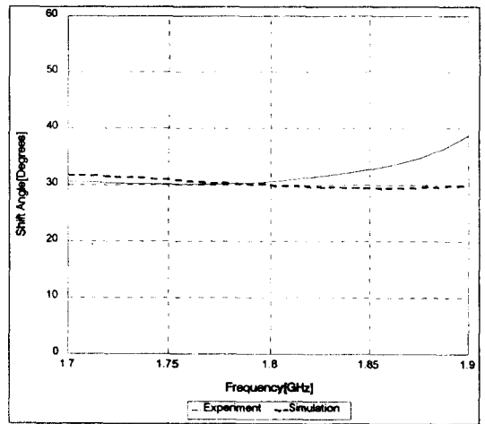
(a) 30° 위상천이기
