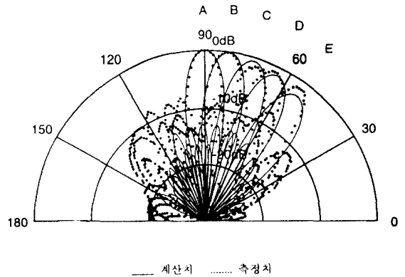
그림 7. 8배열 슬롯결합 위상배열안테나의 방사패턴(계산치, 측정치)
