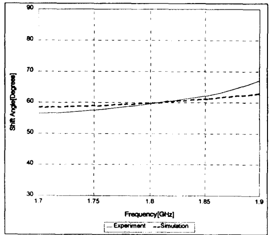
(b) 60° 위상천이기
