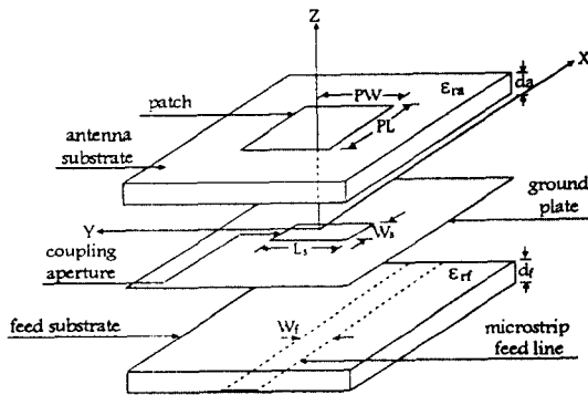
그림 2. 슬롯결합 마이크로스트립 안테나의 구조 Fig. 2. Configuration of a slot coupled microstrip antenna
