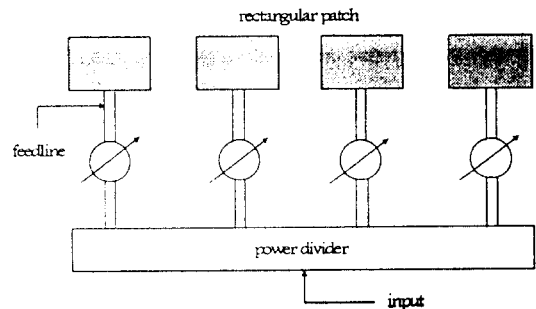
그림 1. 마이크로스트립 위상배열안테나 Fig. 1. Microstrip phased array antenna
