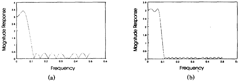
그림 2. 5:3 변환용 실계수 필터의 주파수 응답 (a)21 탭 (b)41 탭
