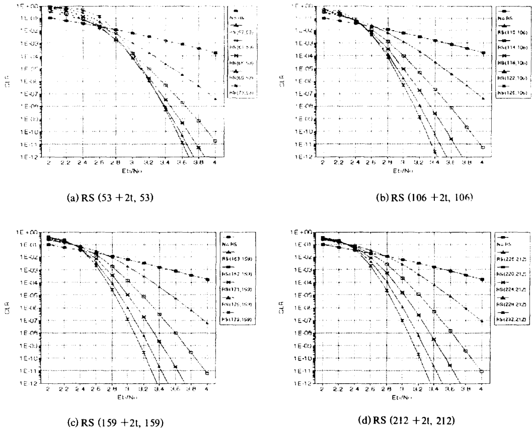
그림 5. 연집에러 환경에서의 기존 53 바이트 ATM 셀의 셀 손실률
