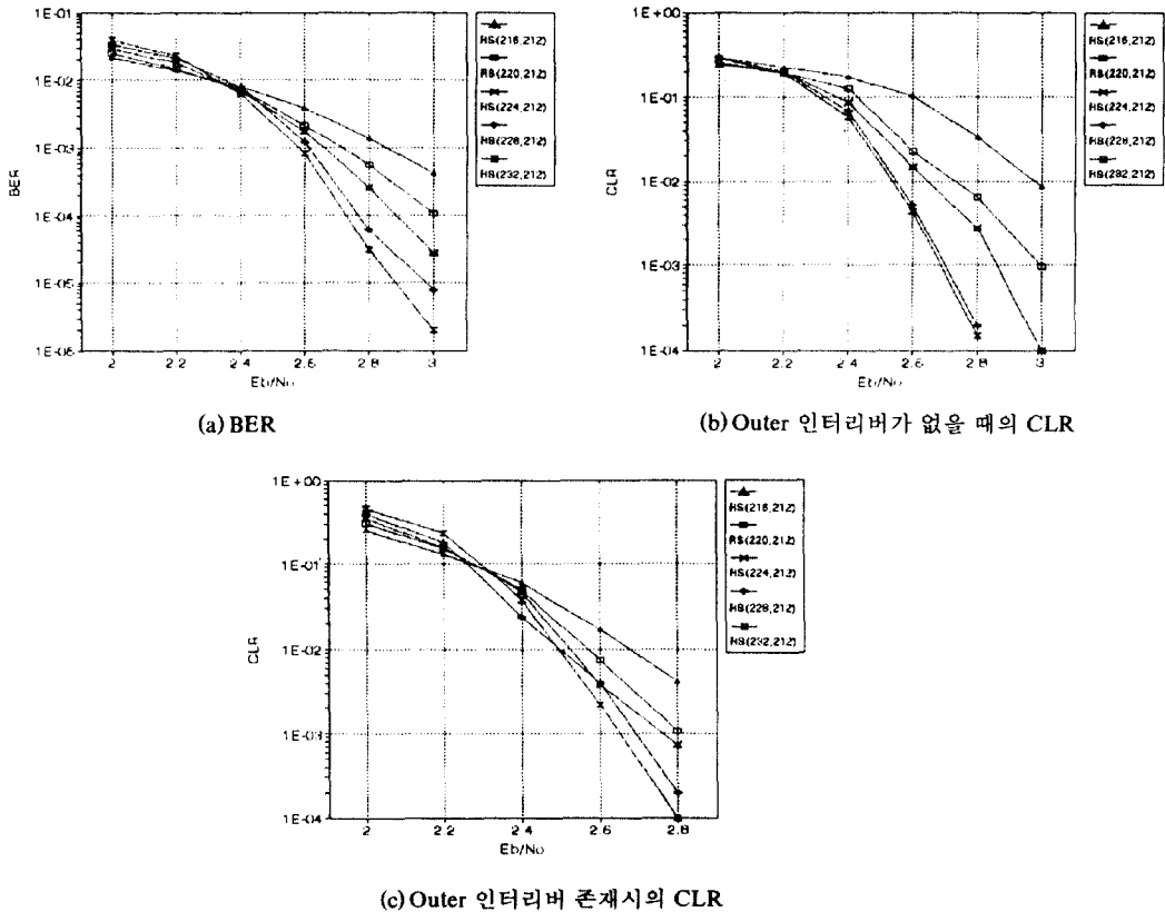
그림 10. 기존의 53 바이트 ATM 셀의 CLR 성능평가
