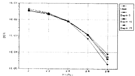
그림 9. Inner 인터리버의 Depth에 따른 BER 성능평가 Fig. 9 BER performances according to Inner Interleaver depth
