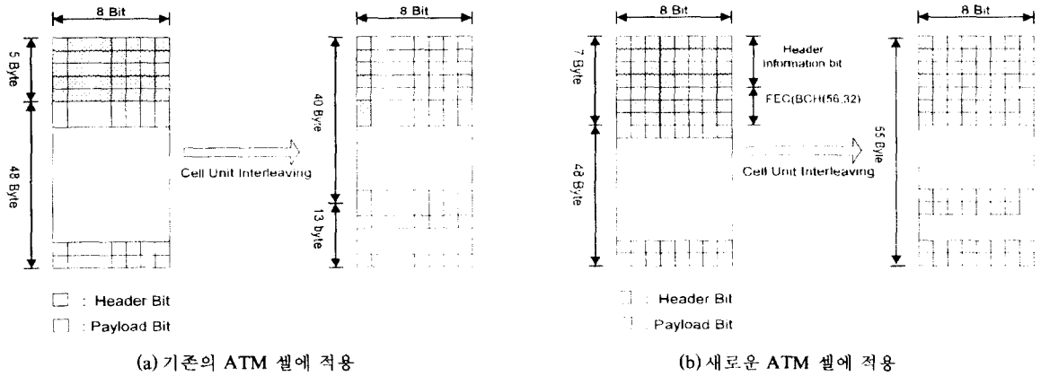
그림 4. CLR 성능향상을 위한 Cell Unit Interleaving 방법
