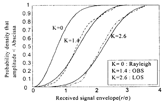
그림 6. LOS와 OBS지역에서의 페이딩 신호와 Rician 파라미터 K의 비교
