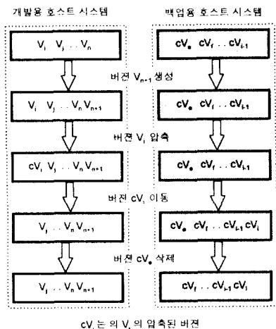
그림 9. CMS-MX 소프트웨어 버전 관리 흐름
