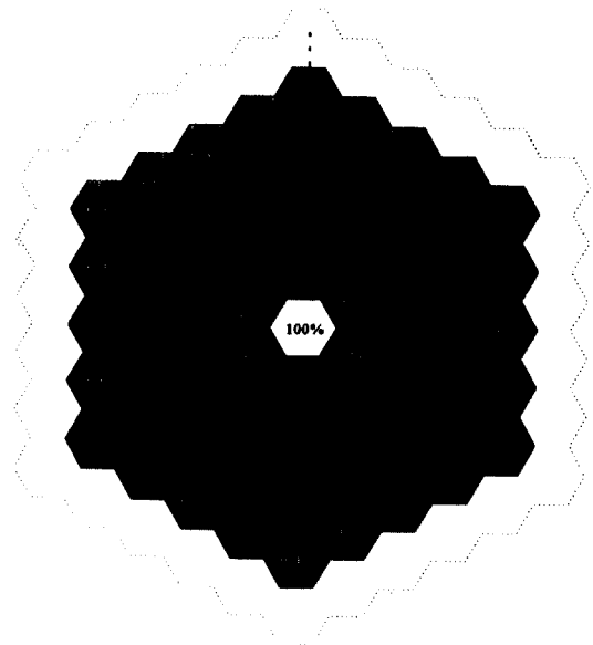
그림 2. 통화량 분포가 균일할 때 인접 셀로부터의 간섭비 파라미터( k_i )의 분포
