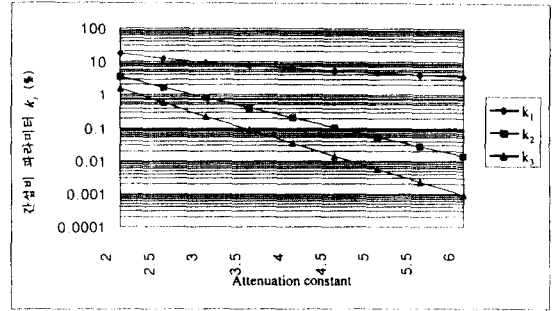
그림 3. 경로 손실에 따른 k_i 의 분포
