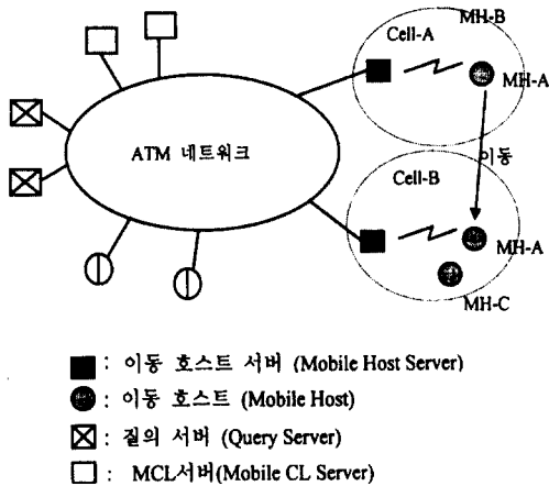
그림1. 이동 컴퓨팅 환경을 위한 네트워크 모델 Fig.1. General network model for mobile computing environments
