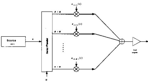
그림 1. Multi-Code CDMA 시스템 전송부
