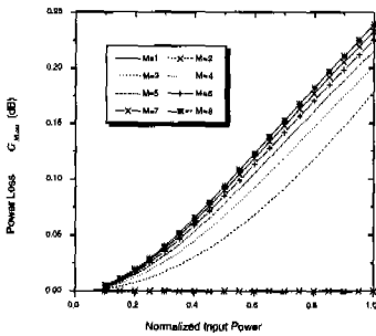
그림 8. 정규화된 입력 전력에 따른 Pdiff의 변화 ( E_b/N_0=10dB , N_b=100 , K=1 , AWGN 채널)
