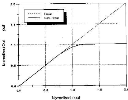
그림 5. 정규화된 전력 증폭기 특성
