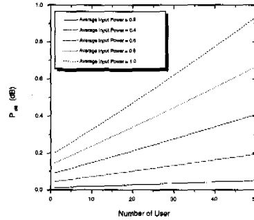
그림 6. 사용자 수에 따른 Pdif의 변화 (Eb/No=10dB, Nb=100, M=4, AWGN 채널)
