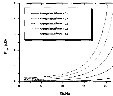
그림 7. Eb/No에 따른 Pdif의 변화 (K=10, Nb=100, M=4, AWGN 채널)
