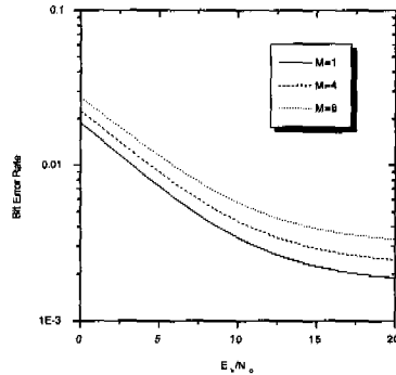
그림 9. BER vs. E_b/N_0 ( K = 20 , N_b=100 , 정규화된 입력 전력 = 1, 주파수 선택적 페이딩 채널)
