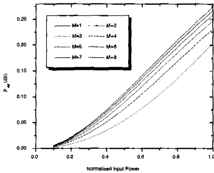
그림 10. 정규화된 입력 전력에 따른 Pdiff의 변화 (Eb/No=10dB, Nb=100, K=1, 주파수 선택적 페이딩 채널)
