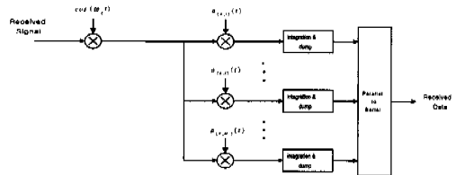
그림 2. 수신기 구조
