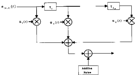
그림 4. 주파수 선택적 페이딩 채널
