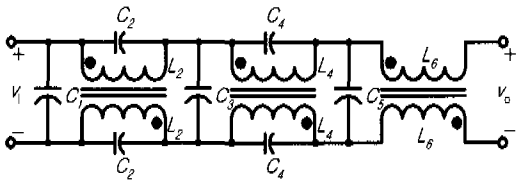
그림 6. 균형 밀결합 변압기를 이용한 지역-통과 여파기.
