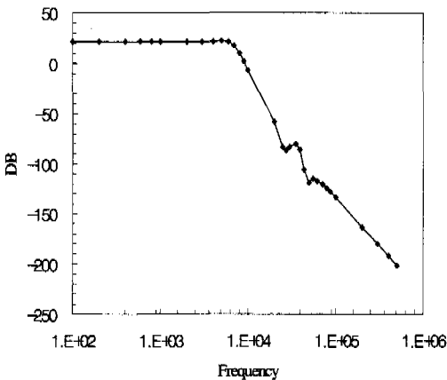
그림 9. 실험에 의한 POTS splitter의 주파수 특성.
