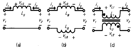
그림 4. 등가 인덕턴스로 나타내기 위한 회로도.
