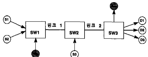
그림 6. 3개의 스위치를 가진 주차장 모델
