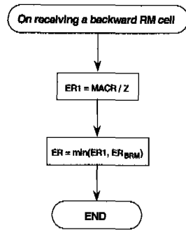
그림 5. 역방향 RM 셀의 처리 루틴
