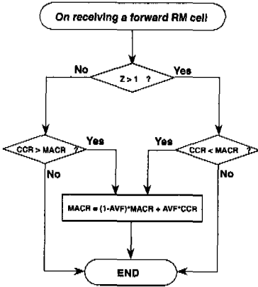
그림 4. 순방향 RM 셀 처리 루틴
