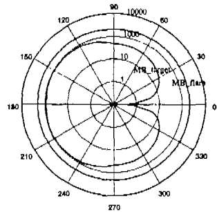
그림 5. 표적 대역에서 방위각에 따른 표적과 섬광탄의 복사 세기
