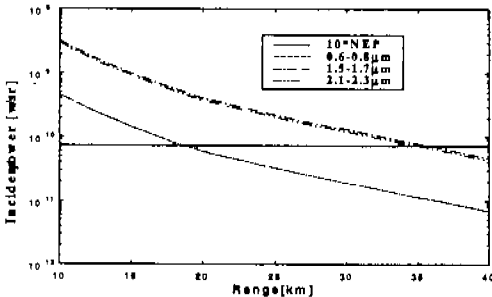
그림 9. 설파광탄의 거리에 따른 입사 에너지
