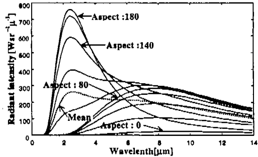
그림 4. 방위각과 파장에 따른 표적의 복사 세기
