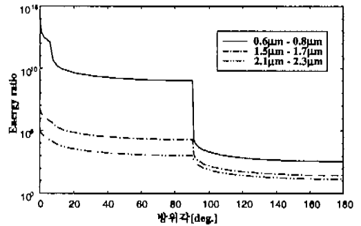
그림 10. 대역에 따른 표적과 설파광탄의 에너지 비
