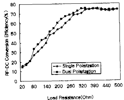
그림 9. 이중편과 정류안테나의 부하에 따른 변환효율(패치)
