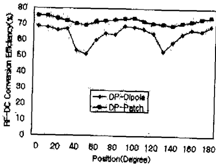
그림 10. 이중편과 정류안테나의 방향에 따른 변환효율
