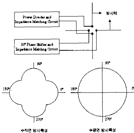
그림 3. 다이폴 형태의 이중편파 정류안테나의 구조와 방사 패턴도
