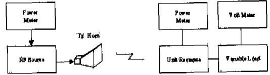
그림 7. 이중편과 정류안테나 변환효율 실험 블록도
