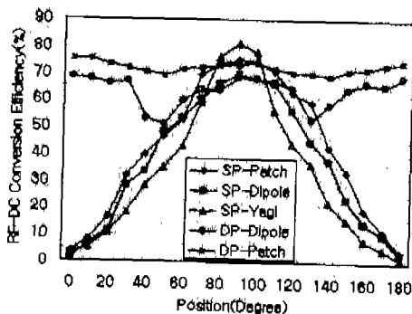
그림 11. 각 정류안테나들의 방향에 따른 변환효율
