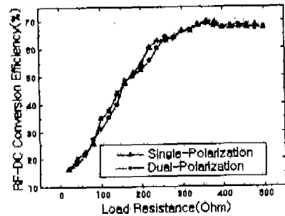
그림 8. 이중편과 정류안테나의 부하에 따른 변환효율(다이폴)
