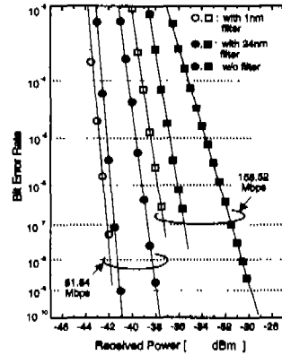
그림 5. 1.5 μm LED 광원의 선폭에 따른 전송성능의 비교
