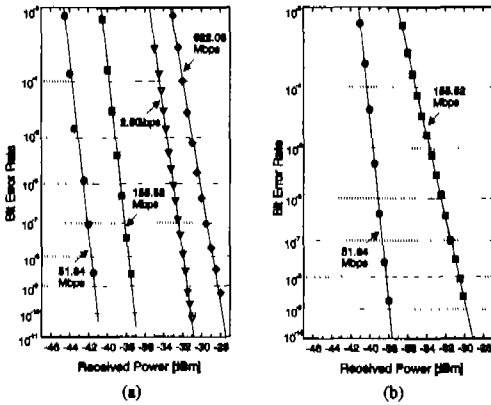
그림 4. 전송성능 측정 결과 (a) 상하향 동시 전송 (하향: 공유레이저 광원 사용, 상향: 1.3 μm LED 사용), (b) 1.5 μm LED를 사용한 상향전송
