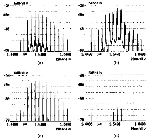
그림 7. 상향전송시의 시스템 포트별 출력 파장 특성 (a) 1.5μm LED 광원만 인가한 경우의 AWG#2 출력 포트 파장성분, (b) 1.5μm LED 및 EDFA의 ASE 신호를 동시에 인가한 경우의 AWG#2 출력포트 파장성분, (c) 1.5μm LED 및 EDFA의 ASE 신호를 동시에 인가한 경우의 AWG#1의 4번 포트 파장성분, (d) EDFA의 ASE 신호만 인가한 경우의 AWG#1의 4번 포트 파장성분
