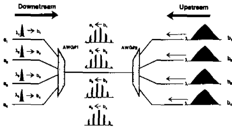
그림 2. WDM-PON 시스템의 광 신호 흐름도
