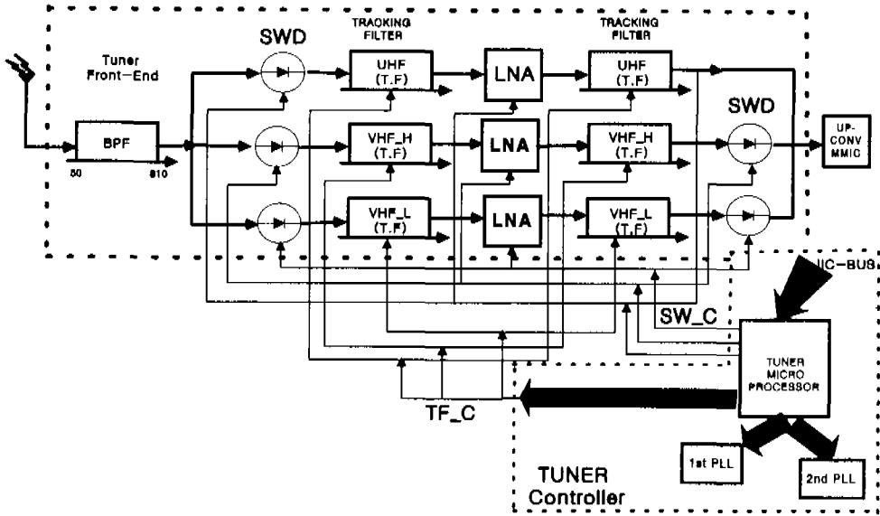
그림 5. 디지털 TV 튜너 전치단 구조도
