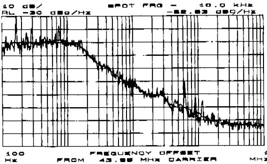
그림 14. 튜너 출력 단의 위상 잡음 (@CH.69)
