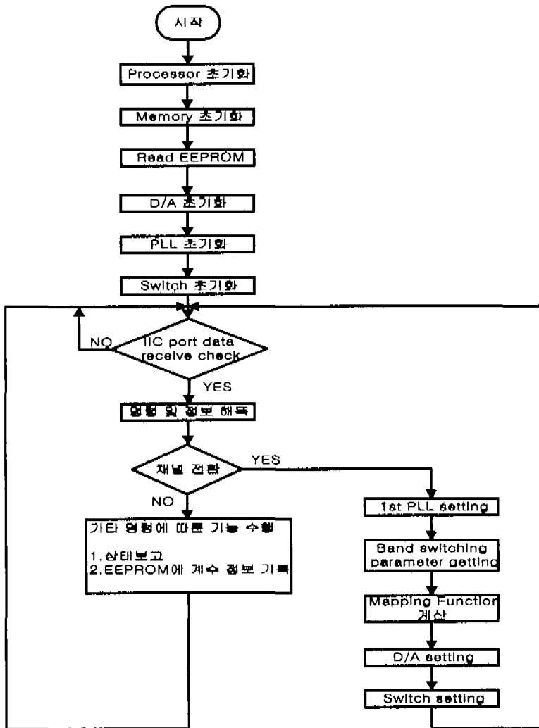
그림 7. 튜너 제어기 신호 흐름도
