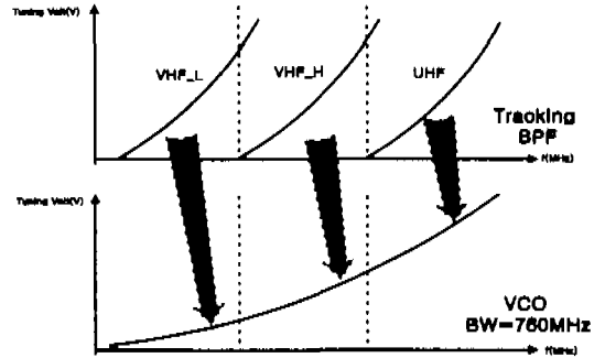
그림 3. 트래킹 필터가 포함된 디지털 TV 튜너 구조의 근사화된 주파수 매핑도
