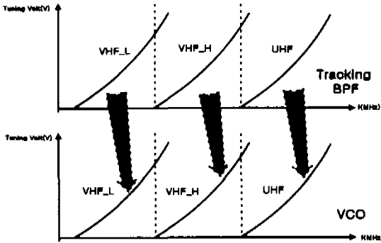
그림 2. NTSC TV 튜너 구조의 근사화된 주파수 매핑도
