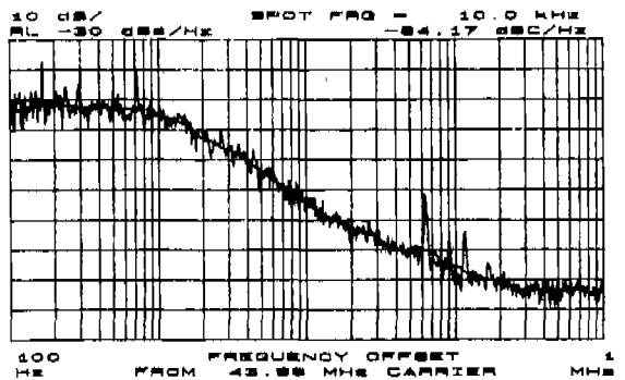
그림 13. 튜너 출력 단의 위상 잡음 (@CH.2)
