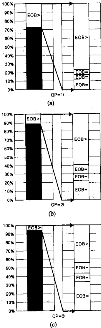
그림 8. Foreman QCIF 동영상에 대한 EOB 값의 분포 (고정된 QP, 30Hz, 300 프레임). EOB 값이 0 이라는 것은 그 블록이 not coded 인을 의미한다.
