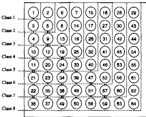
그림 6. DCT 뒤로 양자화된 88 블록의 분류도. 동그라미 속의 숫자는 zig-zag 스캔 순서를 나타낸다. 만약 DCT 및 양자화 후 0이 아닌 계수가 모두 i \times i 사각형 이내에 존재 한다면, 주어진 블록은 class i 로 분류된다.
