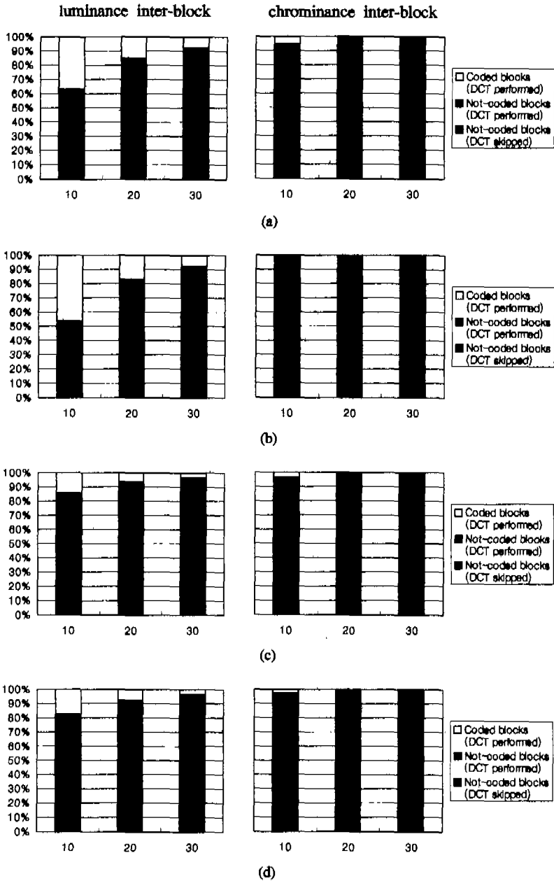
그림 5. DCT 및 양자화를 수행하기 전에 미리 'not coded block' 을 예측한 결과. 가로축 방향의 숫자는 QP를 의미하며 검은 색 막대가 'not coded block' 으로 예측된 부분을 나타낸다.
