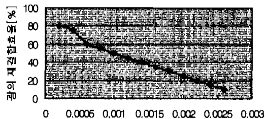
온도에 따른 굴절률변화 dn/dT [^{\circ}\text{C}^{-1}] 그림 7. 열광학효과에 의한 굴절률 변화에 따른 광의 재결합효율
