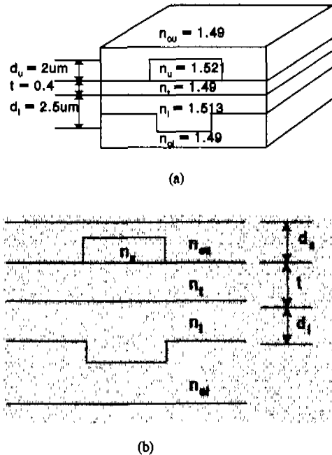
그림 1. 제안된 수직형 광 결합기의 도파로 구조 (a) 전체유체도 (b) 단순화된 2차원 굴절률 분포를 고려한 단면도
