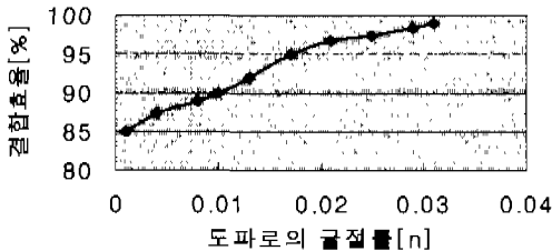
그림 3. 다양한 도파물질 선정에 따른 광 결합도
