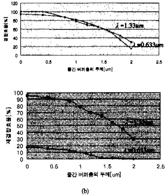
그림 2. 중간 버퍼층 두께에 따른 결합 및 재결합 효율
