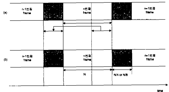
그림 5. 본 논문에서 제안된 frame구조
