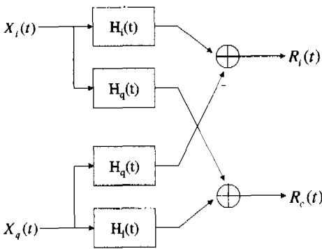
그림 4. Complex baseband system 구조
