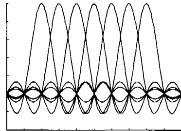
그림 2. OFDM의 부반송파 스펙트럼
