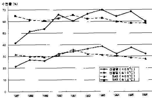
그림 6. 수렴오차 \pm 0.5^{\circ}\text{C} , \pm 1^{\circ}\text{C} 일 때 시계열예측과 예측시 스템의 각 연도별 수렴률
