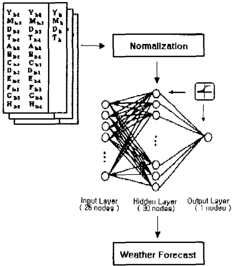
그림 3. 기후예측을 위한 신경망 모델
