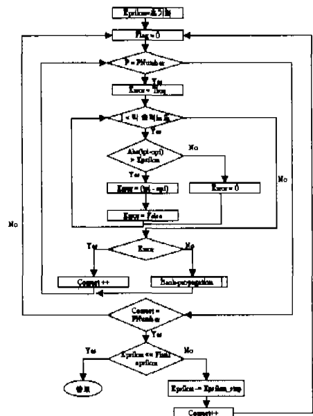
그림 1. Descending Epsilon 알고리즘
