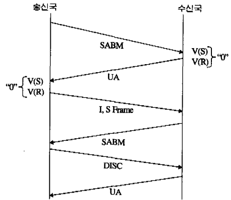
그림 15. AX.25 링크프로토콜 절차
