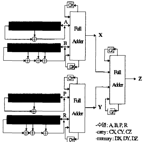
그림 7. 비선형 키수열 발생기
