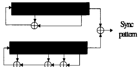
그림 4. 골드코드 구조
