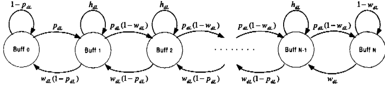
그림 5. 저속 데이터서비스의 마코비안 모델
