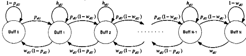
그림 4. 고속 데이터서비스의 마코비안 모델
