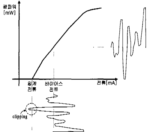
그림 2. LD의 전류에 대한 출력 광전력 곡선
