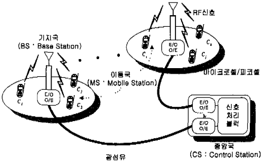
그림 1. CDMA RF 신호전송을 위한 SCM 광링 구조
