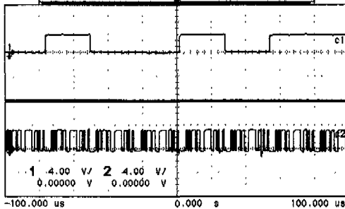
그림 9. 첫 번째 가입자의 신호와 PN 시퀀스의 패턴
