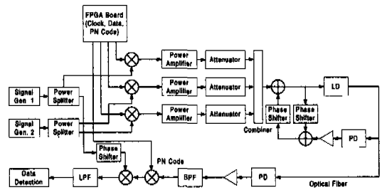
그림 7. 보상구조를 적용한 실험셋업
