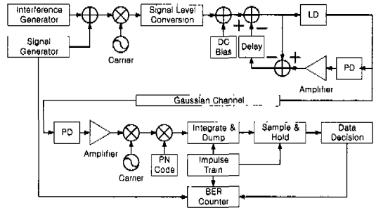
그림 4. LD의 보상구조를 적용한 시뮬레이션 구조
