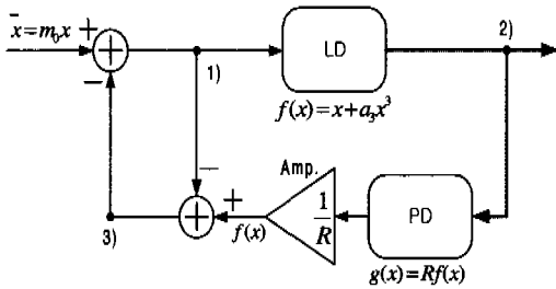
그림 3. LD의 비선형 왜곡 보상구조
