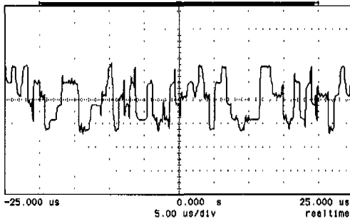
그림 10. 3명의 가입자 신호의 합
