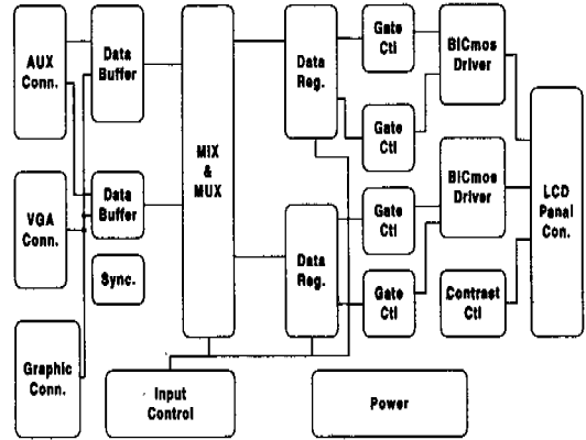
그림 1. Color TFT LCD Driver 블럭도
