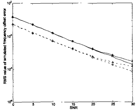
(a) 주파수 오프셋 추정 에러
