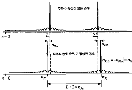
그림 4. 주파수 오프셋이 발생한 수신신호와 동기신호의 상관함수 피크 발생 이동
