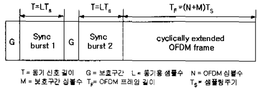
그림 3. 주파수 오프셋 추정 및 프레임 동기를 위해 제안된 OFDM 동기신호 구성
