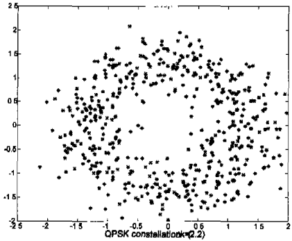
(b) 주파수 오프셋 \Delta k=2.2 인 경우
