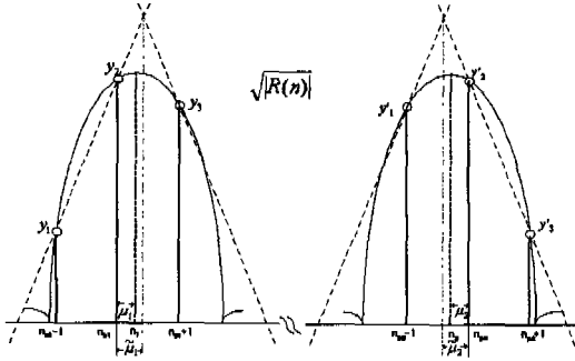
그림 5. 상관함수 최고치 추정 방안
