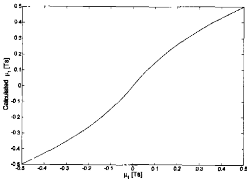
그림 6. \tilde{\mu}_1 와 \mu_1 의 차이 ( T_s=1/8000[\text{sec}] , \Delta\omega=4000[\text{Hz}] , L=400 , \theta_k=4.3 )
