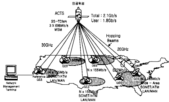
그림 1. ACTS 기가비트 위성통신망 구성도
