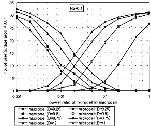
그림 3. 매크로셀에 대한 마이크로셀의 전력비에 따른 outage율 ( R_u=0.1 )
