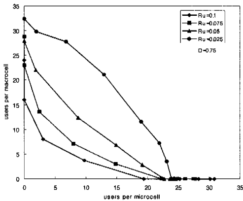
그림 9. 마이크로셀 반경에 따른 용량평면도(D=0.75)
