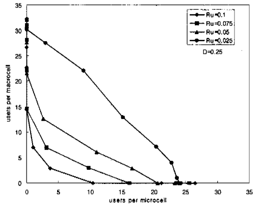
그림 8. 마이크로셀 반경에 따른 용량평면도(D=0.25)
