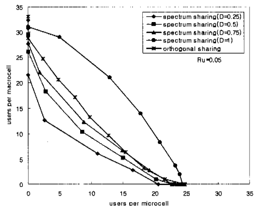
그림 12. 자원 공유 방식의 용량 비교(Ru=0.05)
