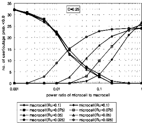
그림 5. 매크로셀에 대한 마이크로셀의 전력비에 따른 outage율(D=0.25)
