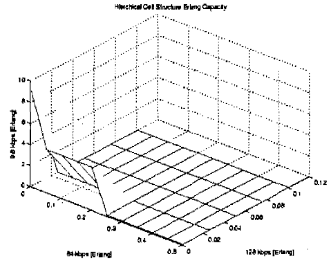
그림 6. 세 종류 서비스를 제공하는 1x 계층셀 시스템의 매크로셀 얼랑 용량(9.6 kbps 음성, 64 kbps 데이터, 128 kbps 데이터)
