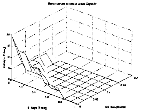
그림 7. 세 종류 서비스를 제공하는 1x 계층셀 시스템의 마이크로셀 얼랑 용량(9.6 kbps 음성, 64 kbps 데이터, 128 kbps 데이터)
