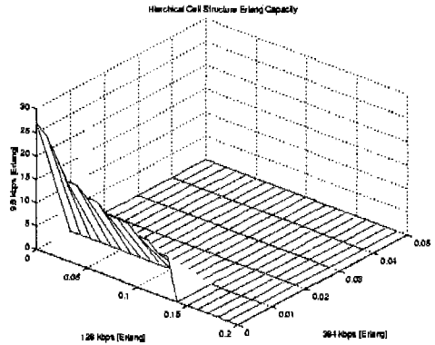
그림 10. 세 종류 서비스를 제공하는 3x 계층셀 시스템의 매크로셀 열량 용량(9.6kbps 음성, 128 kbps 데이터, 384 kbps 데이터)
