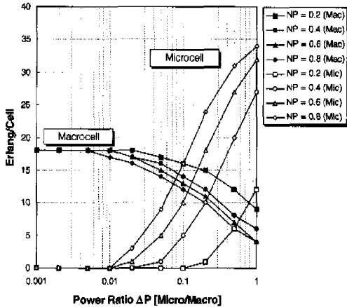
그림 5. 대역 공유 계층셀 시스템의 순방향 용량 (전력 제어 어러 2.5dB, 9.6kbps 음성서비스)
