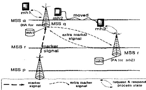
그림 4. 이동하는 mh의 상태 저장
