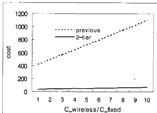
그림 8. C_{wireless} / C_{fixed} 에 따른 통신 비용
