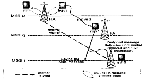
그림 5. 이동성을 고려한 조정된 체크포인트 알고리즘
