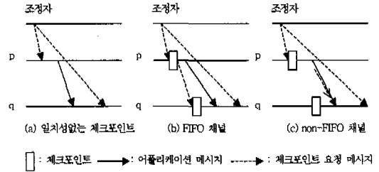
그림 2. 조정된 비블럭킹 체크포인팅 (Nonblocking coordinated checkpointing)
